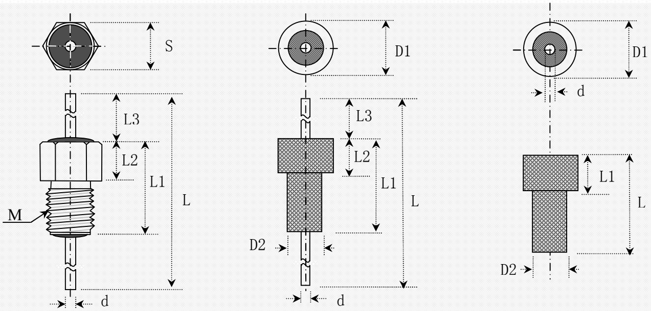
螺纹式
